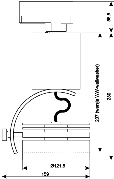
Wymiary w milimetrach
