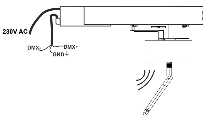
PX795 w trybie odbiornika
