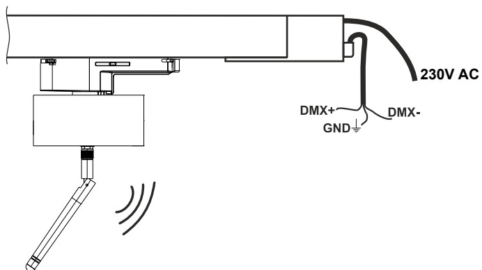
PX795 w trybie nadajnika
